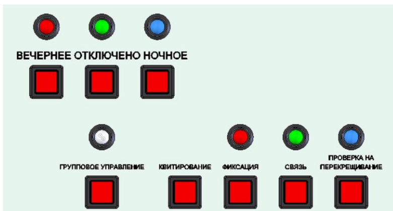
Рис. 6. Панель группового управления ПУ.
