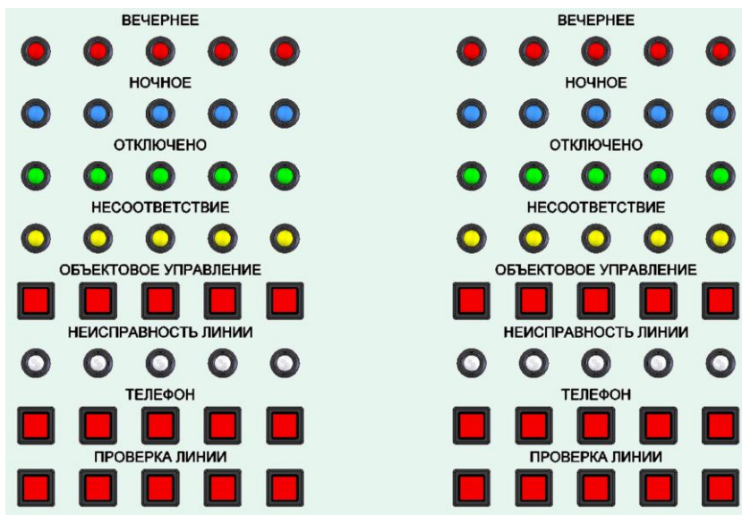
Рис. 5. Панель объектового управления ПУ.
